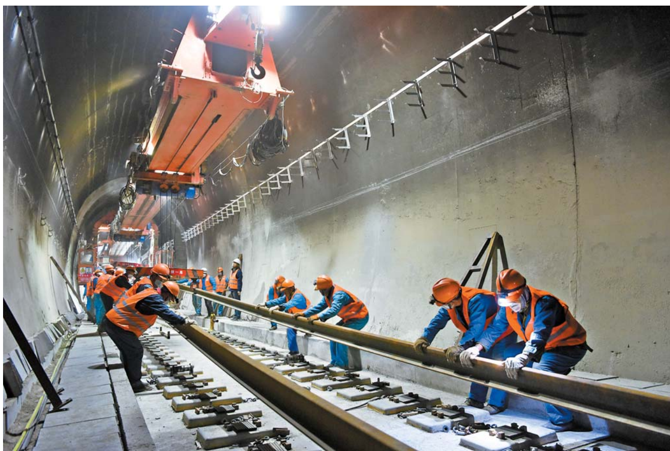
5 - ئاينىڭ 29 - كۈنى، ئىشچىلار ئالتۇنتاغ تونېلى ئىچىدە رېلىس ياتقۇزماقتا. شۇ كۈنى، گولمۇد - كورلا تۆمۈريولى(شىنجاڭ بۆلىكى)دىكى ئەڭ ئۇزۇن تونېل — ئالتۇنتاغ تونېلىدا رېلىس ياتقۇزۇش ۋەزىپىسى تاماملاندى.
